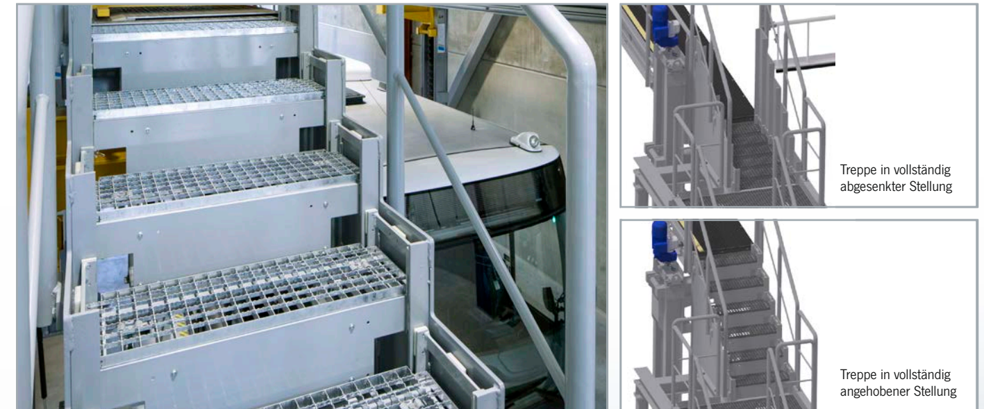
Verstellbare Treppe mit korrekter Stufenhöhe: Führt den Mitarbeiter sicher an den Arbeitsplatz.
